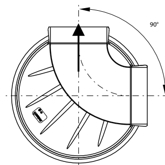
Bodem met stroomprofiel bocht 90°
